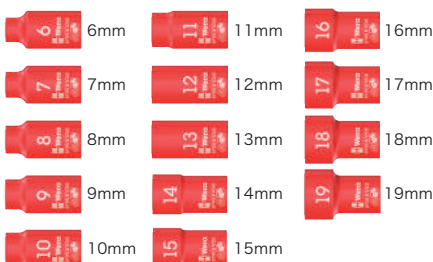
絶縁ソケット(差込角3/8")
