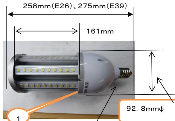
外形寸法
