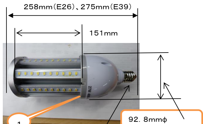
外形寸法
