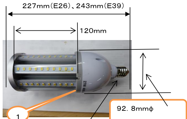
外形寸法
