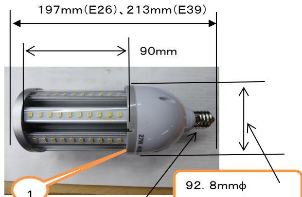
外形寸法
