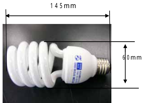
外形寸法
