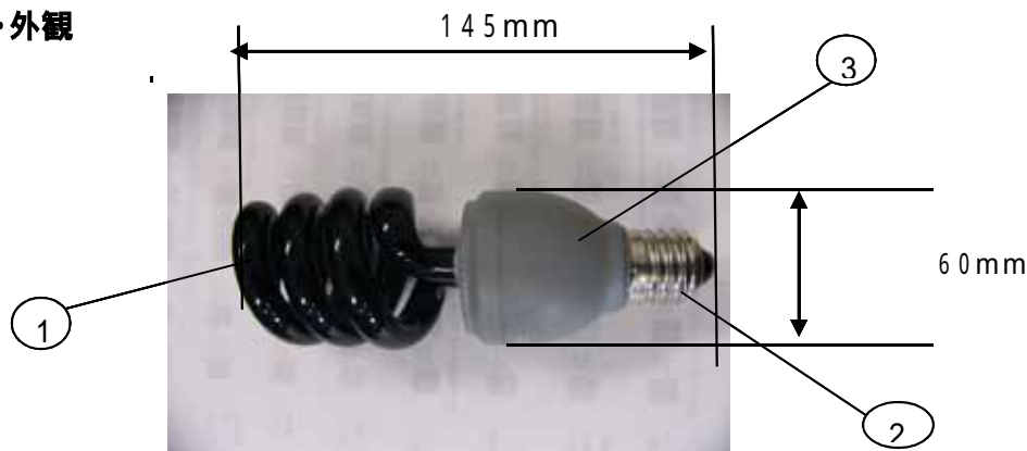
外形寸法
