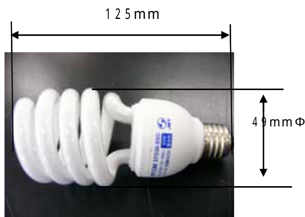
外形寸法
