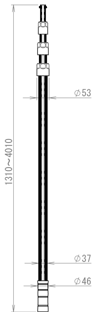
アルミポール4.0m DLC-AP40S
