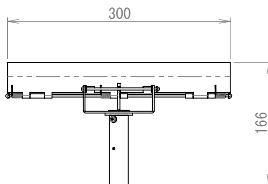
クランプヘッド DLC-RT
