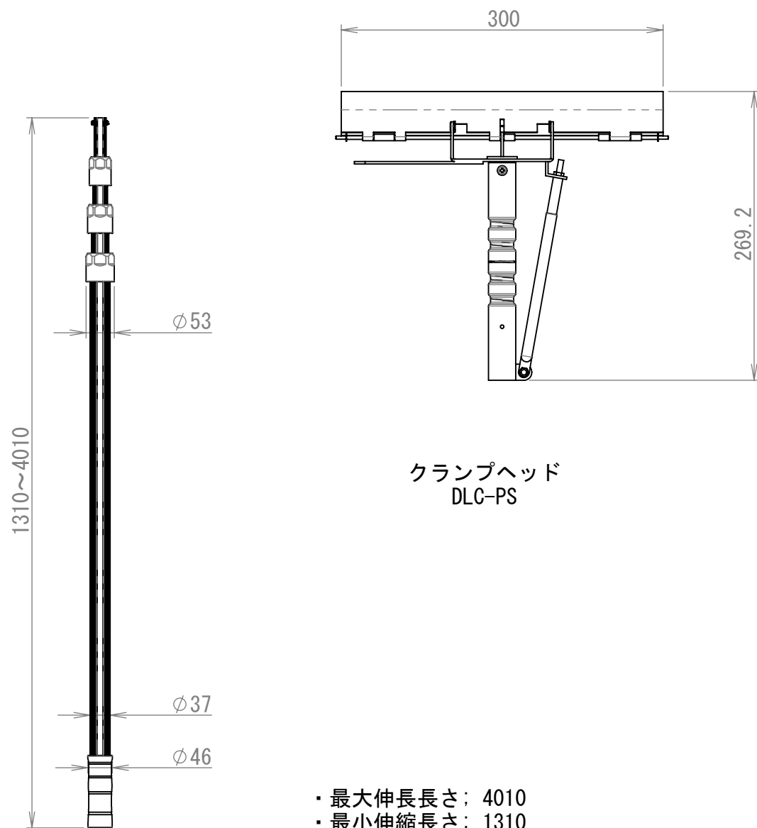
アルミポール4.0m DLC-AP40S
