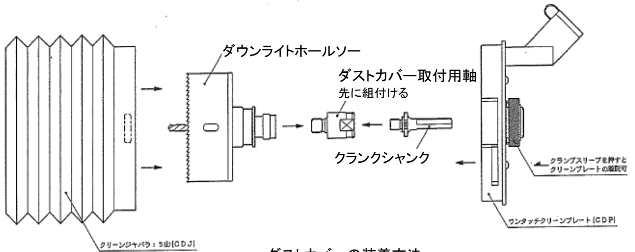
ダストカバーの装着方法
