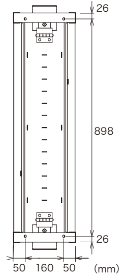
■連結用穴位置【図2】 (下から見た図)
