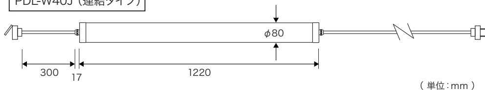
PDL-W40J (連結タイプ)
