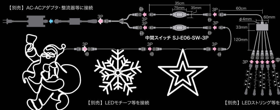
中間スイッチ SJ-E06-SW-3P 5分岐コード SJ-E06-B05
