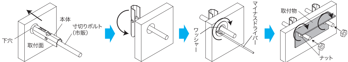
AP-9N(ボルトなしタイプ)
