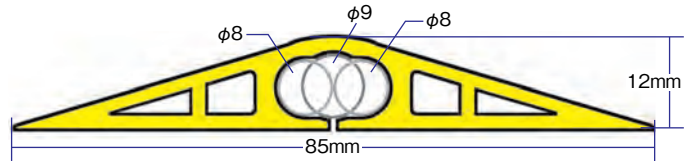
SFM-8509 【適応電線類】 ケーブルφ9mm以下、5C2V(2本)、 VVF 2.0×3C、VVF 2.6×2C
