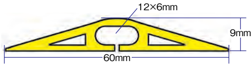
SFM-6006 【適応電線類】 電話線、通信線、ビニール平形コード、 VVF 1.6×2C
