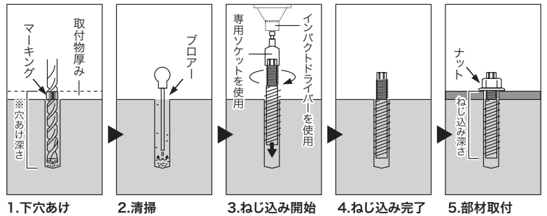
1. 下穴あけ ※埋込深さ+10mm +取付物厚み
