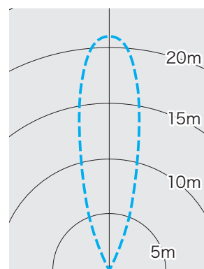
PDS-C02-40FL(集光型)
