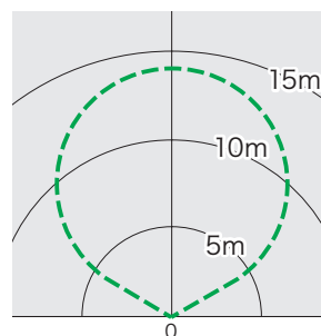
PDS-C01-40WL(散光型)
