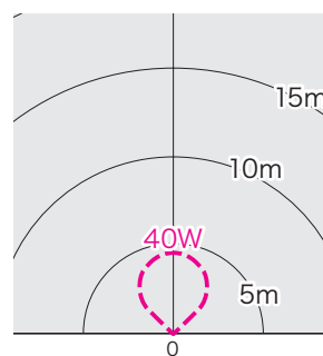
PDS-C01-40FL (40W型)
