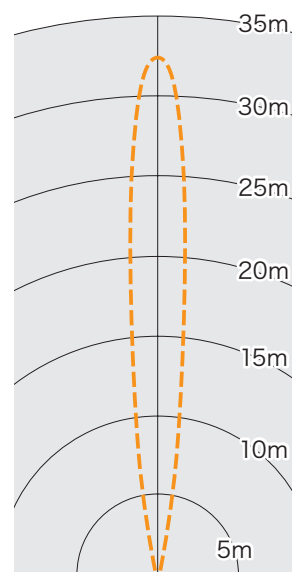
PDS-C02-40WL(集光型)
