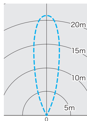
PDS-C02-40FL(集光型)
