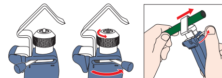
レバー操作で刃の向きを90°変え、電線に沿って縦方向に被覆をカットできる
