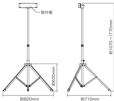
取付け板 PD-32F
